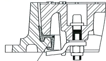
PORMENOR - B (Fecho de segurança)
