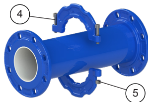
Flange passa-muros ajustável de DN 50 a DN 200
