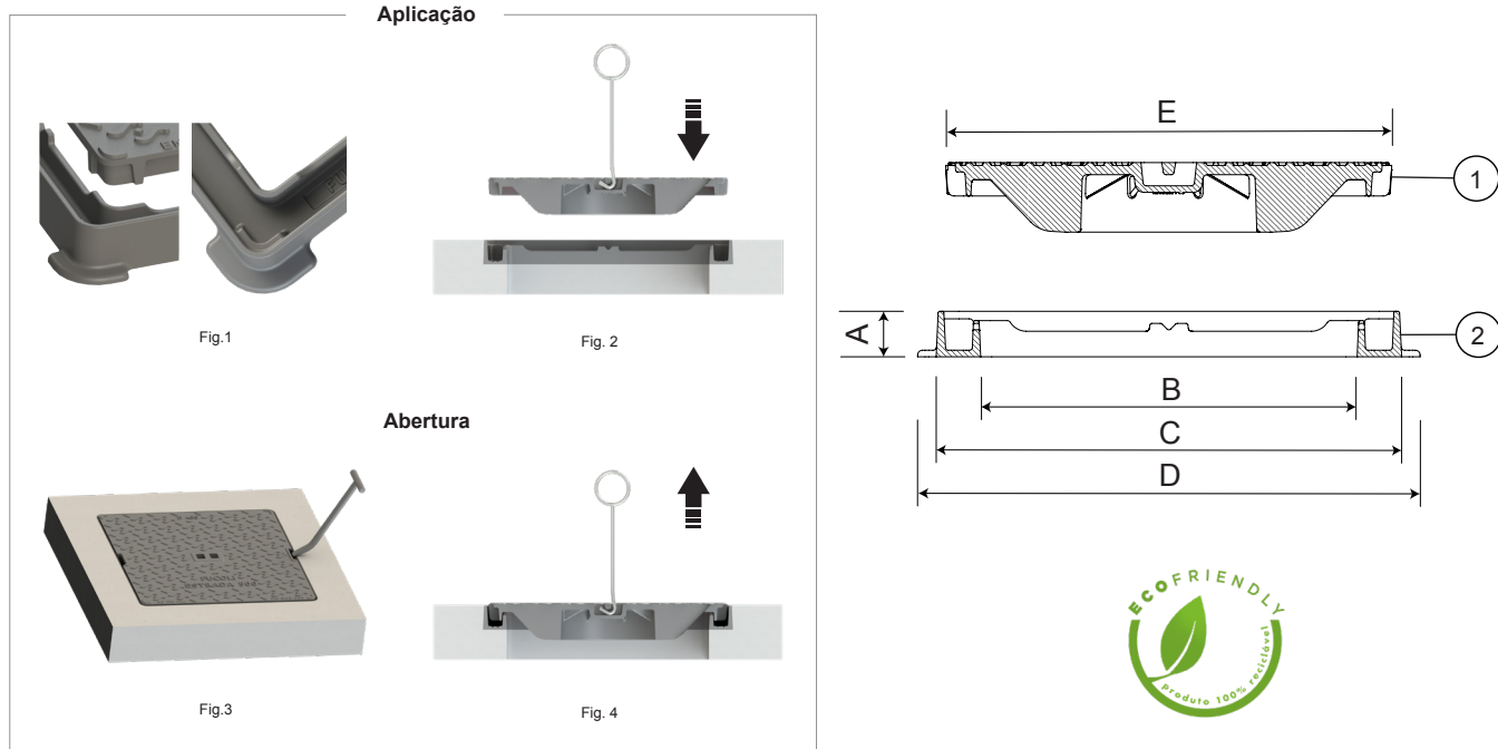
Fig.1 - Sistema de encaixe antirruído
