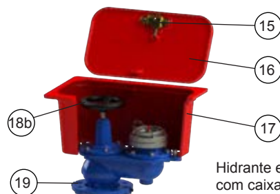
Hidrante enterrado com caixa de proteção opção com dado
