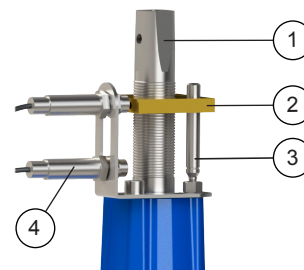
Pormenor do indicador de posição e fins de curso
