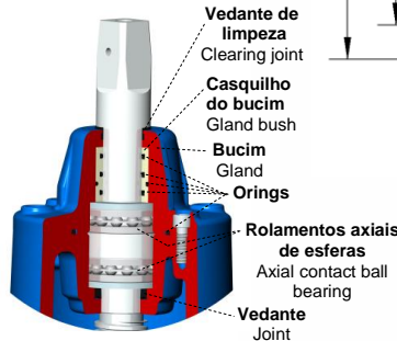
Válvulas de cunha elástica de DN350 a DN500 Soft sealing gate valve DN350 up to DN500
