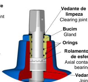
Válvulas de cunha elástica de DN250 a DN300 Soft sealing gate valve DN250 up to DN300
