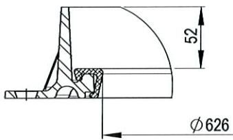
Pormenor - B Apoio Elástico
